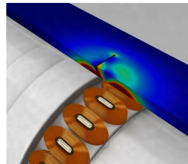
Sonde CF multiéléments flexible
