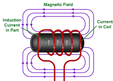
Banc de Magnétoscopie, Machine de soudage, de chauffage/trempe par induction
